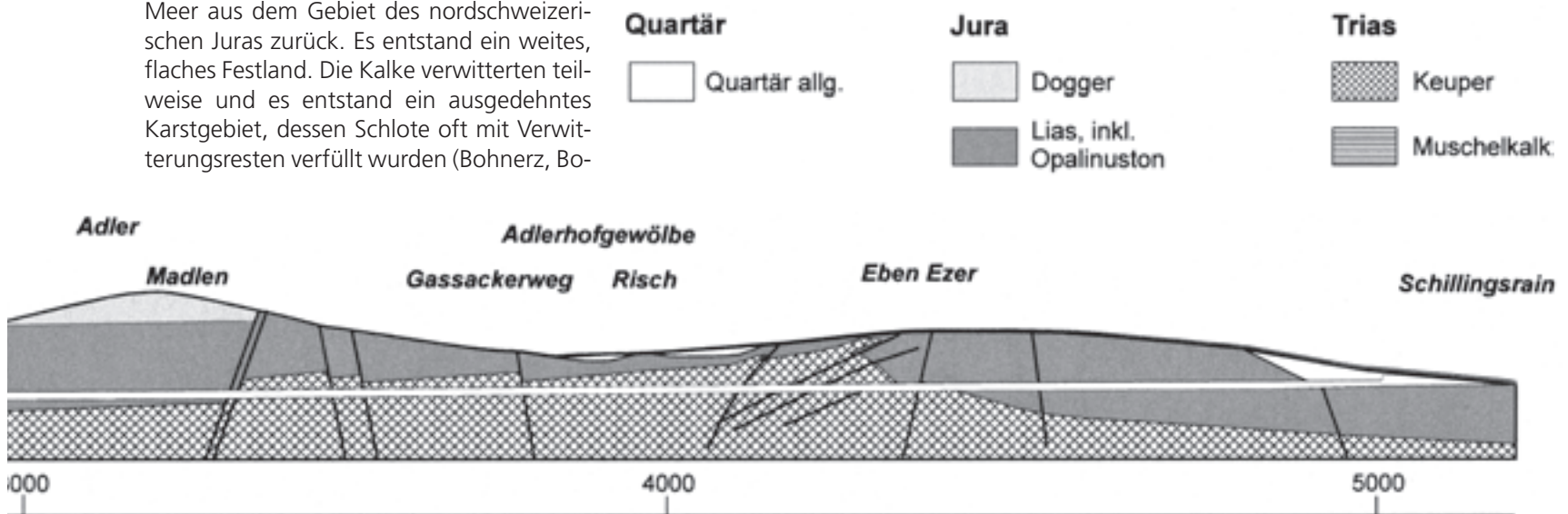
Abb. 2: Geologisches Längsprofil des Adlertunnels, erstellt und 2003 zur Publikation freigegeben durch Martin Meyer, Dipl. Geologe, Geotechnisches Institut AG, Basel.
